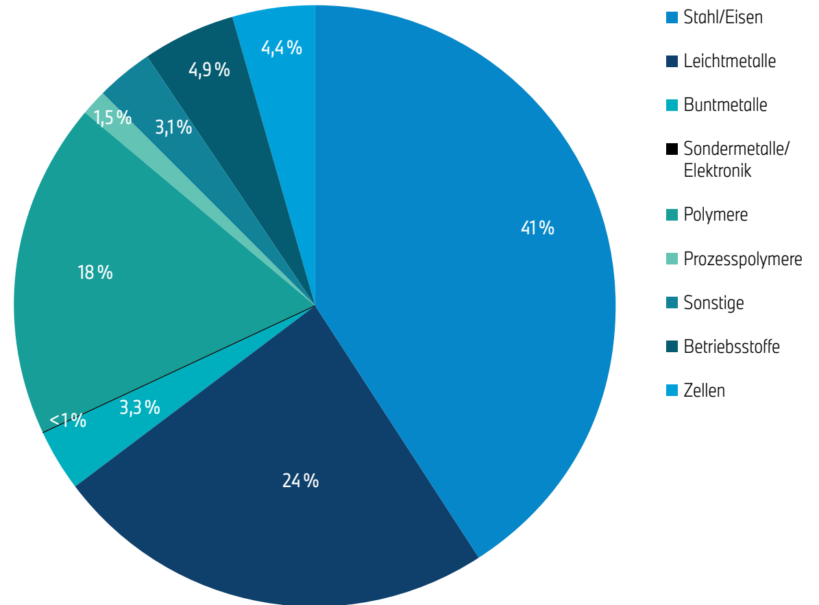
Abb. 2: Werkstoffzusammensetzung des BMW 530e Touring zum Produktionsstart. Die angegebenen Werte können Rundungsdifferenzen aufweisen.
